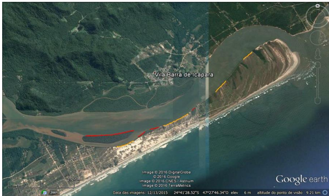
Figura 3.2.2.4.4-2 – Áreas erodidas em manguezal (vermelho) e praia arenosa (laranja), na região da ARIE do Guará.
